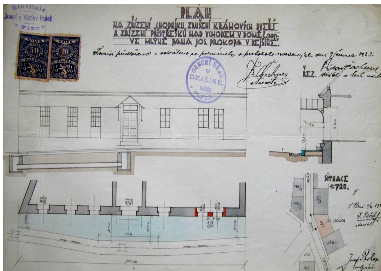
Stavební výkres r. 1923 (stav. arch.)
