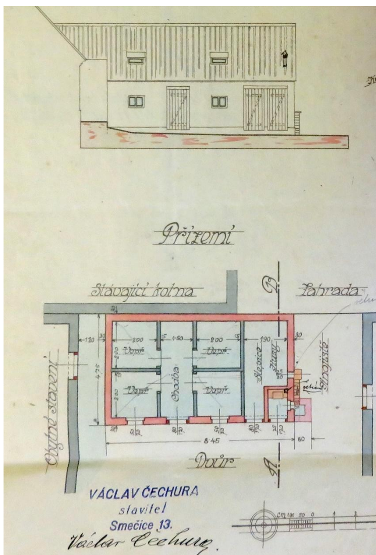
Výkres pro povolení stavby chlívků Martina Štrunce 1920 (stav. arch.)
